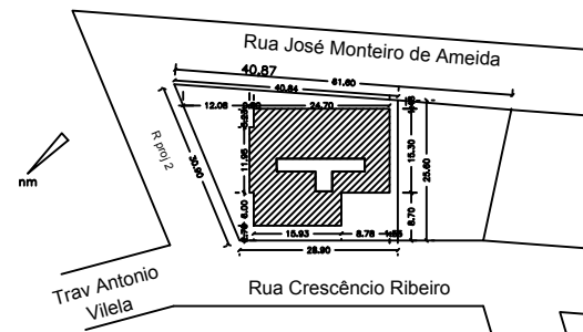
PLANTA BAIXA ESC.: 1:250
