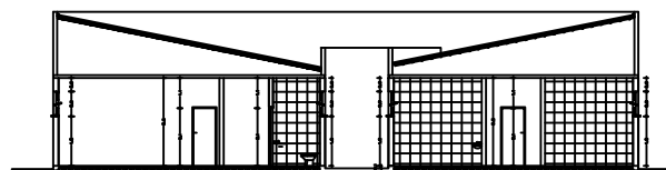
CORTE BB, Esc 1:100
